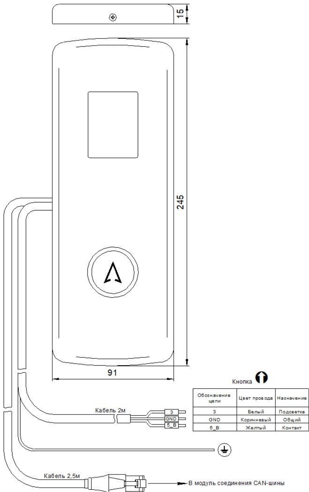
Рис.1 Внешний вид, габаритные и установочные размеры Вызывного поста ЦИРКОН (жгут RJ45) НШЕК.468381.035
